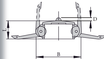
QCDC DC Dust Cap
